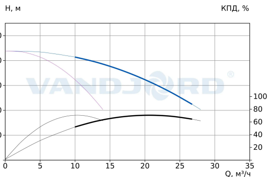
75211425 Hydro-FS-A 2/1 CRV 10-4 G2-B-80-16
