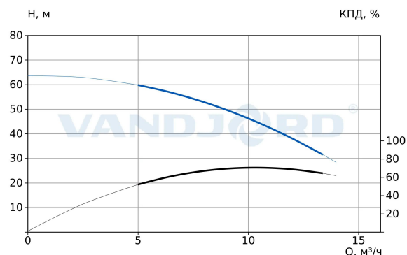
75211389 Hydro-FS-A 1/1 CRV 10-6 G2-B-80-16
