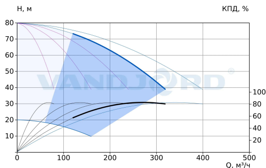
75111511 Hydro-ME 5 CRVE 64-3-1 G2-B-D-250-16-A
