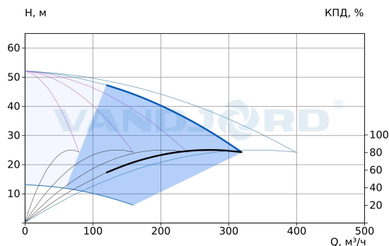
75111508 Hydro-ME 5 CRVE 64-2-1 G2-B-D-250-16-A
