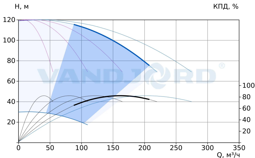
75111503 Hydro-ME 5 CRVE 45-5-2 G2-B-D-200-16-A
