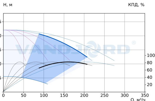
75111495 Hydro-ME 5 CRVE 45-1-1 G2-B-D-200-16-A
