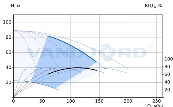
75111489 Hydro-ME 5 CRVE 32-5-2 G2-B-D-150-16-A
