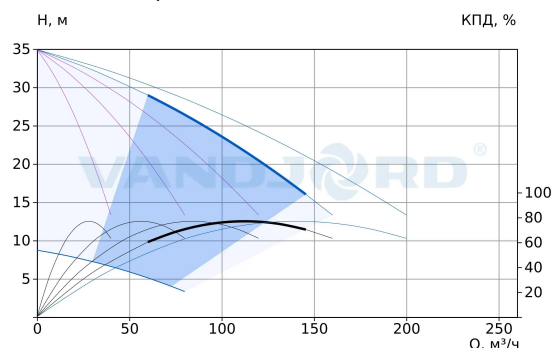
75111483 Hydro-ME 5 CRVE 32-2-2 G2-B-D-150-16-A
