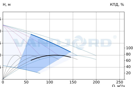
75111482 Hydro-ME 5 CRVE 32-1 G2-B-D-150-16-A
