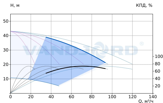
75111464 Hydro-ME 5 CRVE 15-3 G2-B-D-150-16-A
