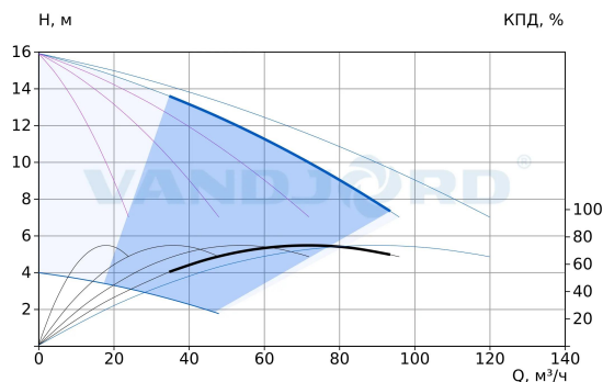
75111462 Hydro-ME 5 CRVE 15-1 G2-B-D-150-16-A
