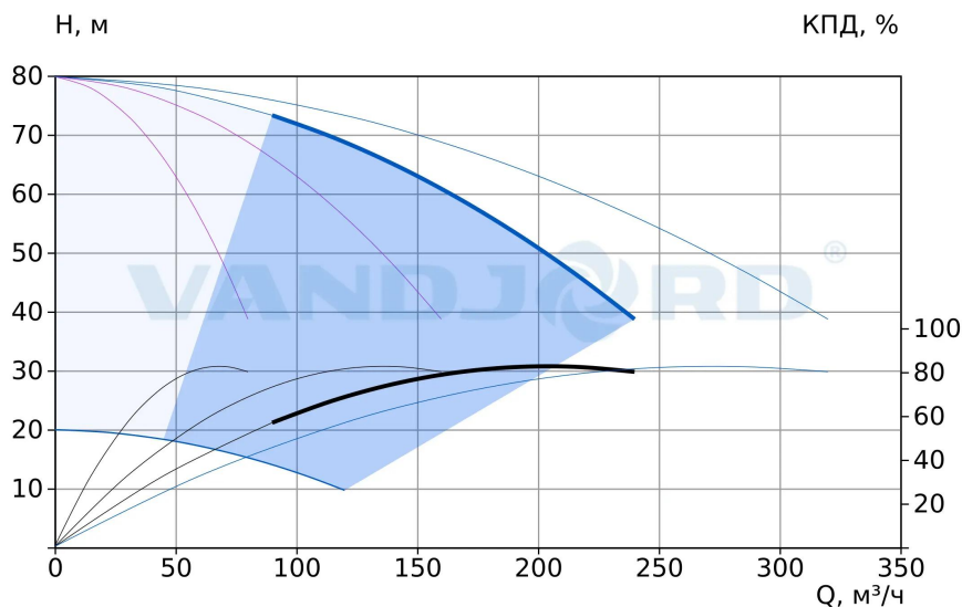
75111398 Hydro-ME 4 CRVE 64-3-1 G2-B-D-200-16-A
