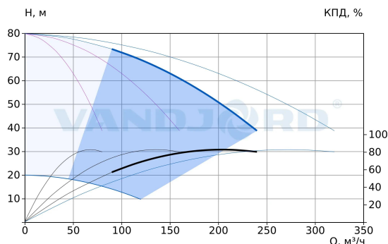
75111398 Hydro-ME 4 CRVE 64-3-1 G2-B-D-200-16-A
