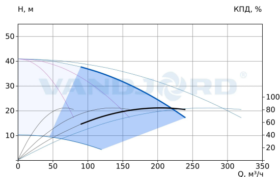
75111395 Hydro-ME 4 CRVE 64-2-2 G2-B-D-200-16-A
