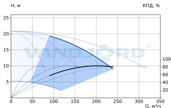
75111393 Hydro-ME 4 CRVE 64-1-1 G2-B-D-200-16-A
