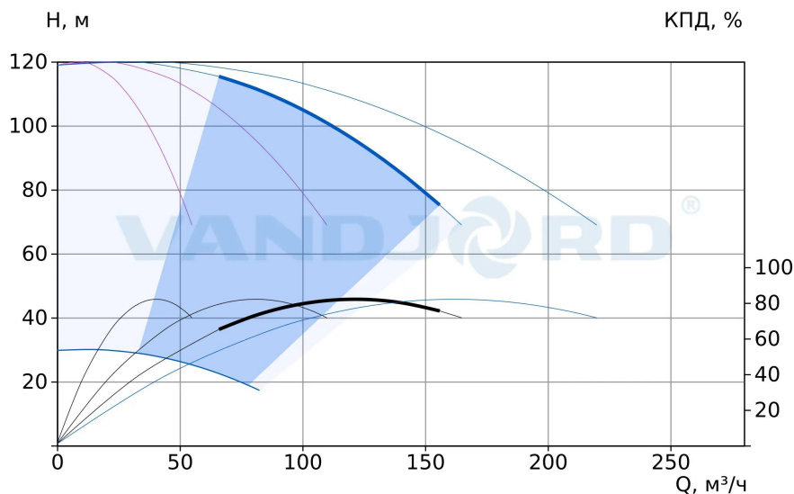
75111391 Hydro-ME 4 CRVE 45-5-2 G2-B-D-200-16-A
