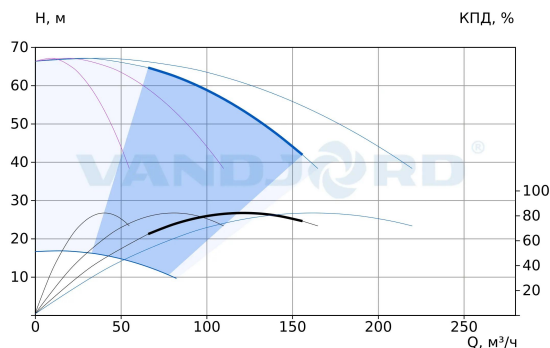
75111388 Hydro-ME 4 CRVE 45-3-2 G2-B-D-200-16-A
