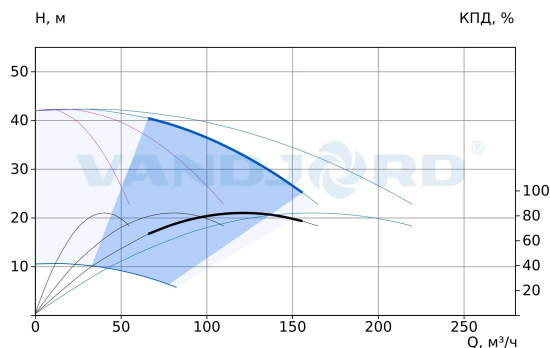
75111386 Hydro-ME 4 CRVE 45-2-2 G2-B-D-200-16-A
