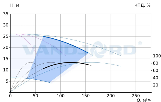
75111385 Hydro-ME 4 CRVE 45-1 G2-B-D-200-16-A
