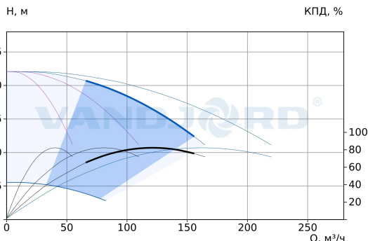
75111384 Hydro-ME 4 CRVE 45-1-1 G2-B-D-200-16-A
