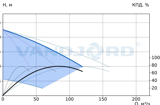
75111371 Hydro-ME 4 CRVE 32-1 G2-B-D-150-16-A
