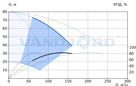
75111178 Hydro-ME 3 CRVE 64-3-1 G2-B-D-200-16-A
