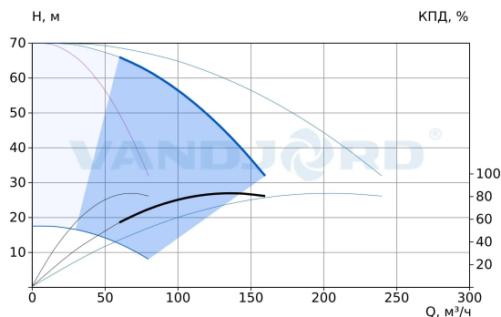
75111179 Hydro-ME 3 CRVE 64-3-2 G2-B-D-200-16-A
