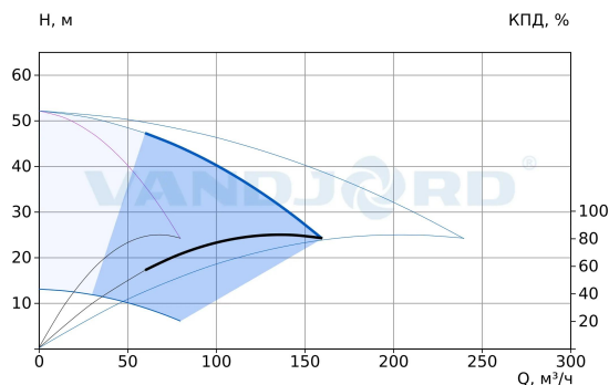
75111290 Hydro-ME 3 CRVE 64-2-1 G2-B-D-200-16-A
