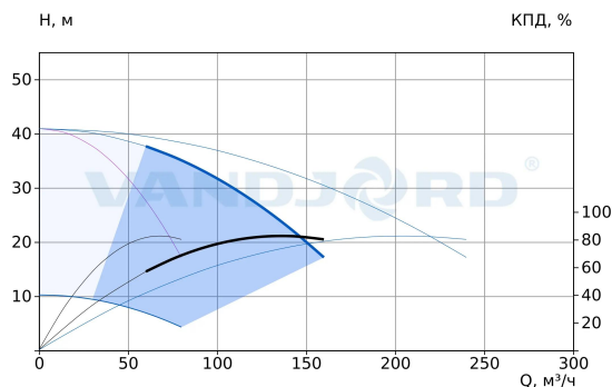
75111289 Hydro-ME 3 CRVE 64-2-2 G2-B-D-200-16-A
