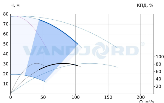
75111093 Hydro-ME 3 CRVE 45-3 G2-B-D-150-16-A
