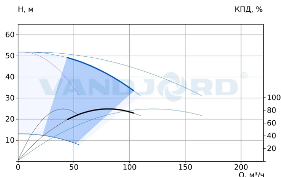
75111186 Hydro-ME 3 CRVE 45-2 G2-B-D-150-16-A
