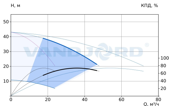
75111066 Hydro-ME 3 CRVE 15-3 G2-B-D-100-16-A
