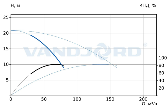
75111235 Hydro-ME 2 CRVE 64-1-1 G2-B-D-150-16-A
