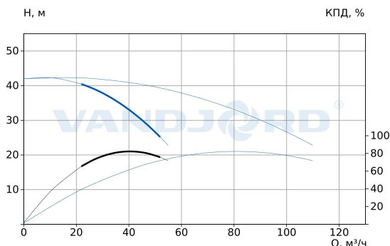
75111087 Hydro-ME 2 CRVE 45-2-2 G2-B-D-150-16-A
