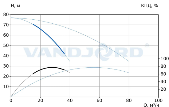
75111081 Hydro-ME 2 CRVE 32-4 G2-B-D-100-16-A
