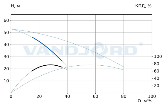
75111222 Hydro-ME 2 CRVE 32-3-2 G2-B-D-100-16-A
