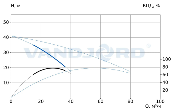
75111221 Hydro-ME 2 CRVE 32-2 G2-B-D-100-16-A
