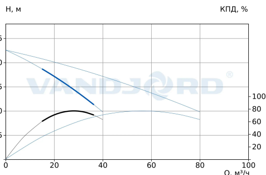
75111220 Hydro-ME 2 CRVE 32-1 G2-B-D-100-16-A
