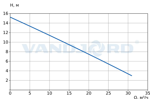
71121014 MEGA S 50-15F 1x230V
