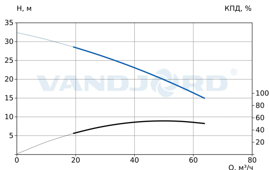
76352012 VSE.80.55.2.C.160.N.5.0D.E
