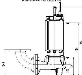
Переносная установка (колено заказывается отдельно)
