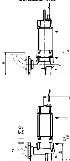
Переносная установка (колено заказывается отдельно)
