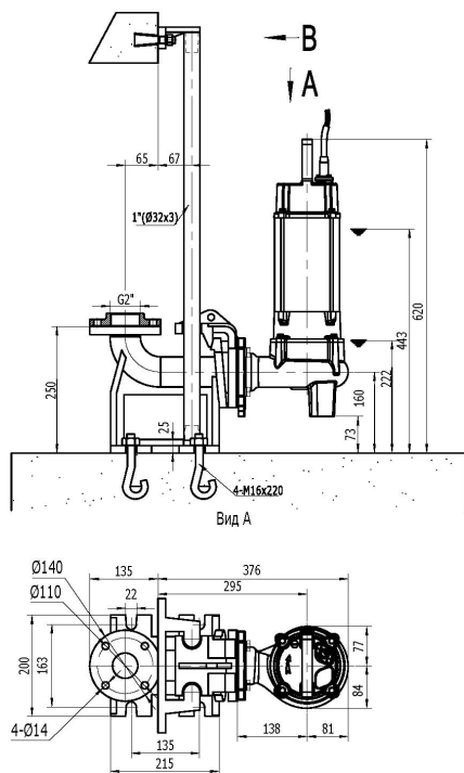
Установка на автоматической трубной муфте
