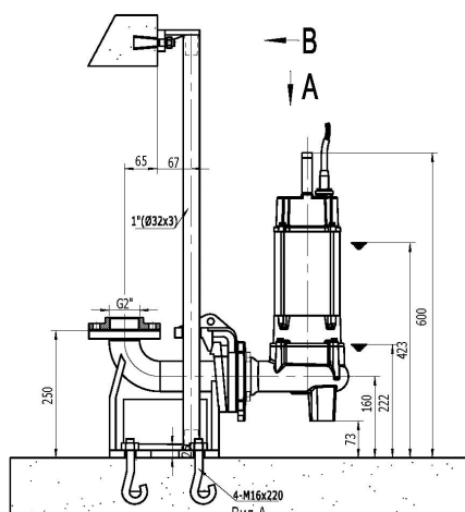
Установка на автоматической трубной муфте
