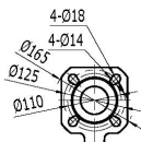
Фланец насоса PN 6/10
