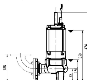
Переносная установка (колено заказывается отдельно)
