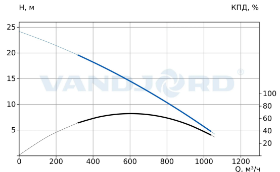
76328002 VSL.300.370.4.5.1D
