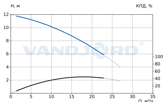
76321710 VSL.50.075.A.2.1.502
