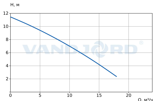
76221306 APV.40.40.08.1.V
