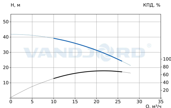
74212027 VCM 20-3C A-R-F-E
