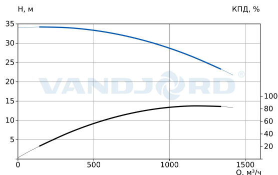
73124104 TPV 350-270-110/4 Q-A-BT-E
