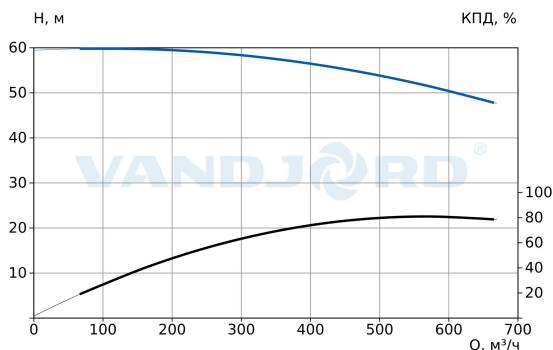
73121139 TPV 200-520-110/4 Q-A-BT-E
