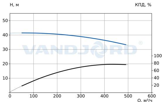
73121136 TPV 200-360-55/4 Q-A-BT-E
