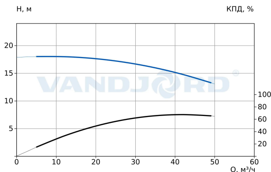
73115134 TPV 65-150-3/4 Q-A-BT-E
