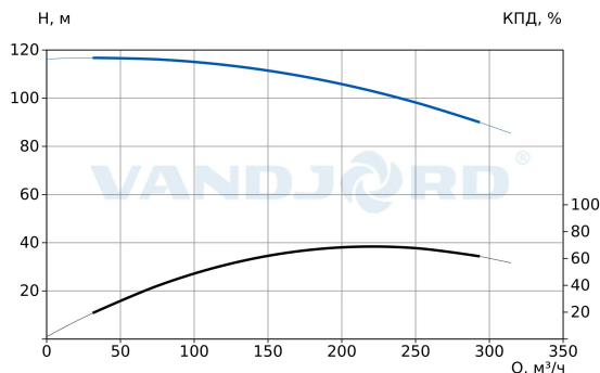
73117147 TPV 100-1020-110/2 Q-B-BT-E
