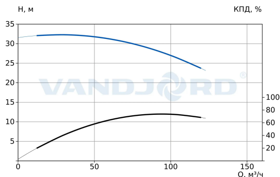
73116134 TPV 80-270-11/2 Q-A-BT-E
