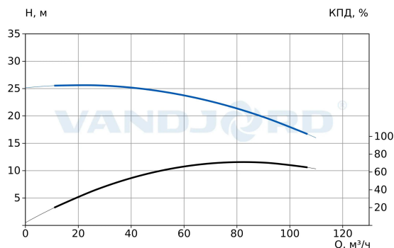
73116133 TPV 80-200-7.5/2 Q-A-BT-E
